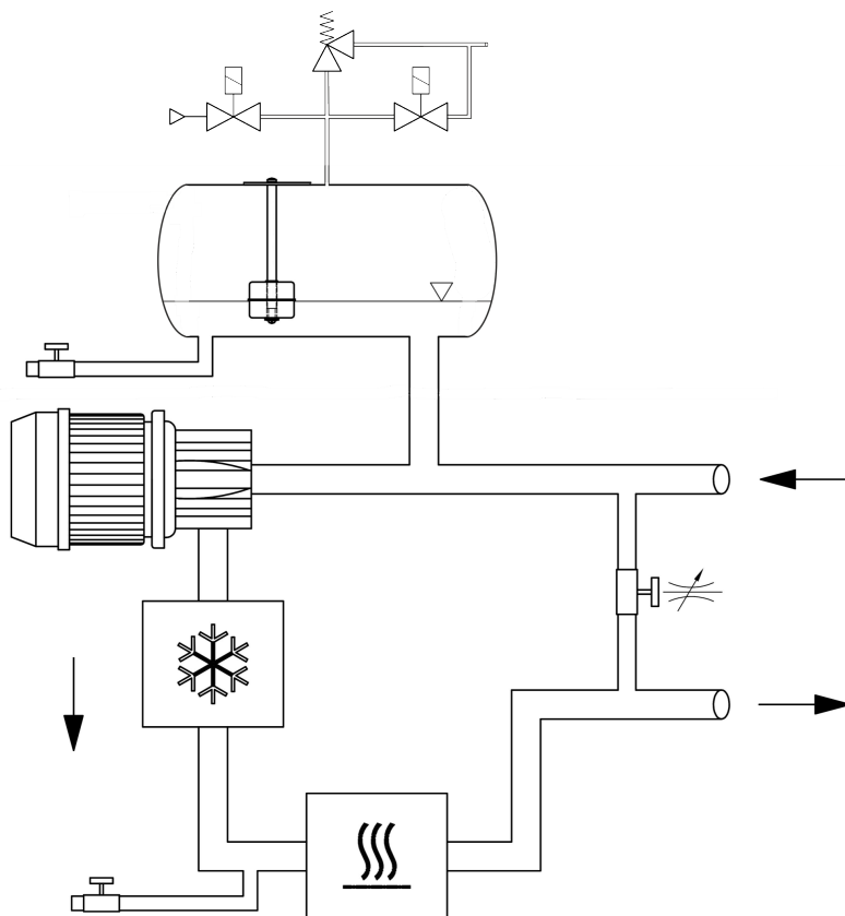
Abb. 9: Schema des Hydraulikkreislaufs bei Geräten IN P
