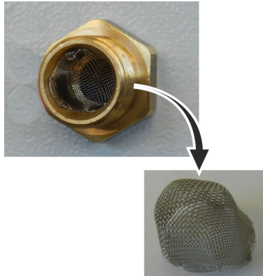
Abb. 93: Filtersieb entnehmen
