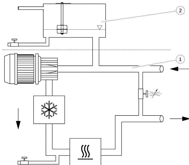
Abb. 8: Schema des Hydraulikkreislaufs bei Geräten IN XT
