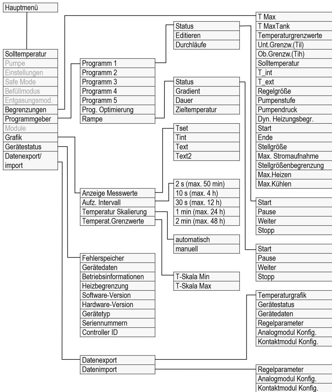
Abb. 39: Menü Teil 3, Fortsetzung von vorheriger Seite
