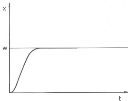
Abb. 78: optimale Einstellung
