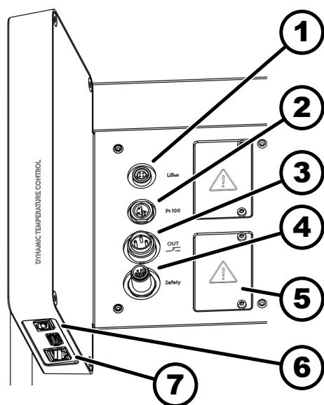
Abb. 11: Schnittstellen
