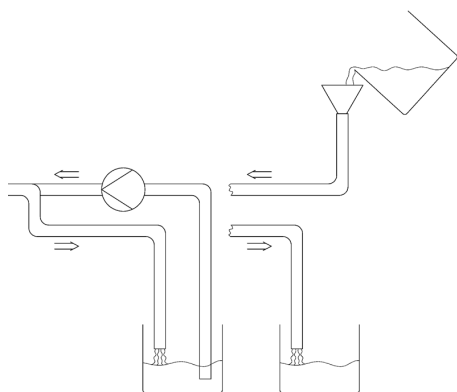
Abb. 94: Entkalken
