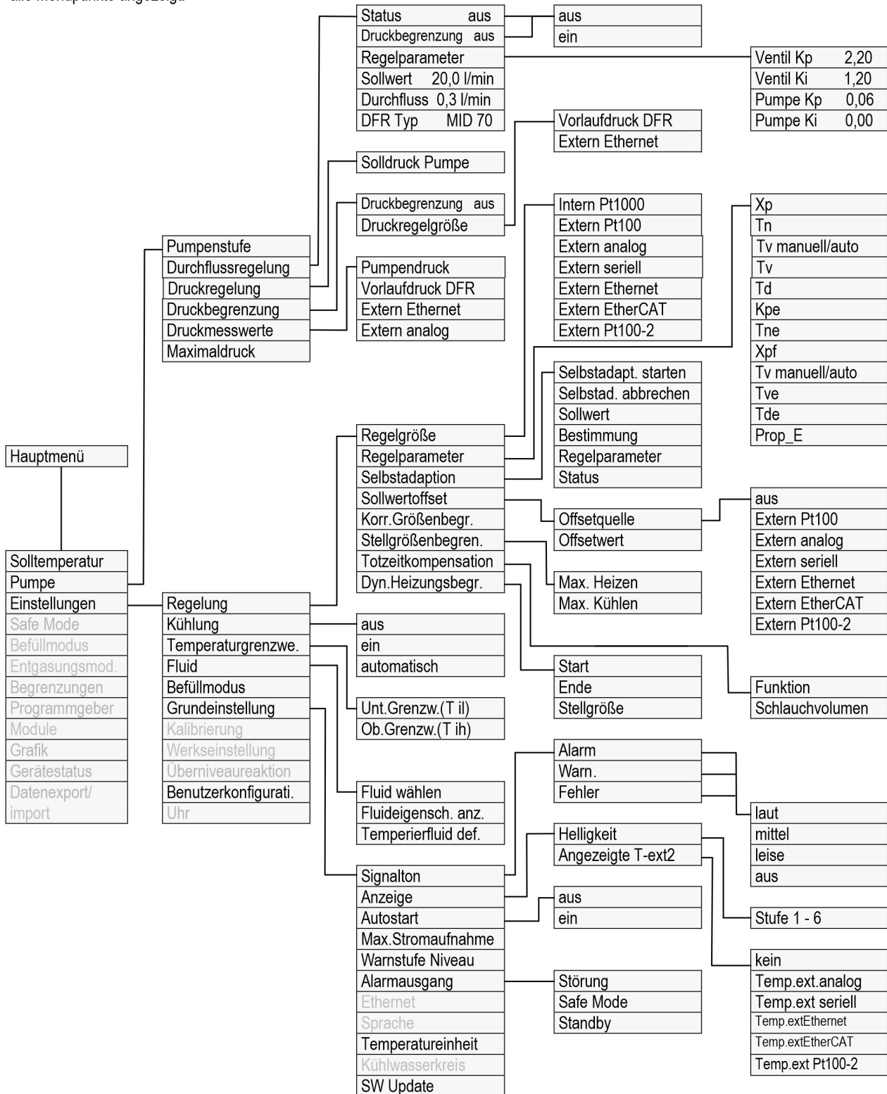
Abb. 37: Menü Teil 1
