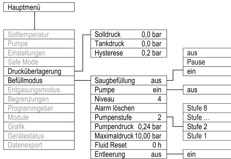
Abb. 40: Menüstruktur der Drucküberlagerung
