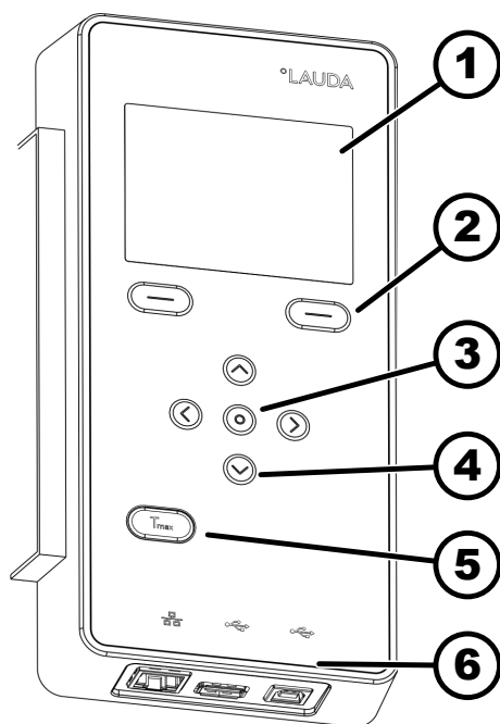
Abb. 28: Bedieneinheit
