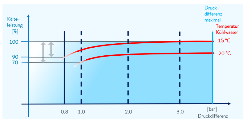
Abb. 99: Druckdifferenz Kühlwasser
