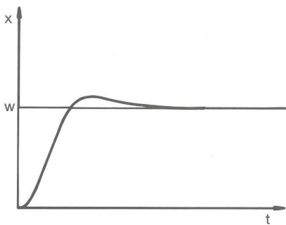
Abb. 79: Regelparameter X_p zu groß
