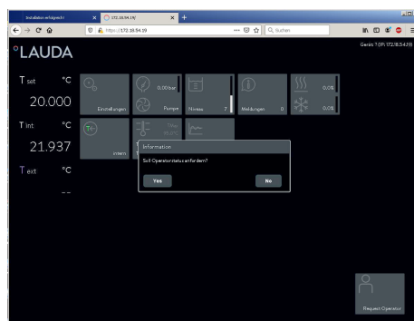
Abb. 86: Webserver im Browserfenster
