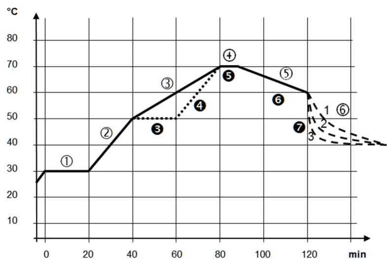
Abb. 62: Programm Beispiel
