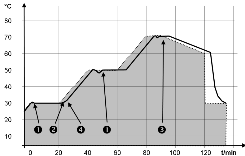
Abb. 63: Programmverlauf Soll-Ist
