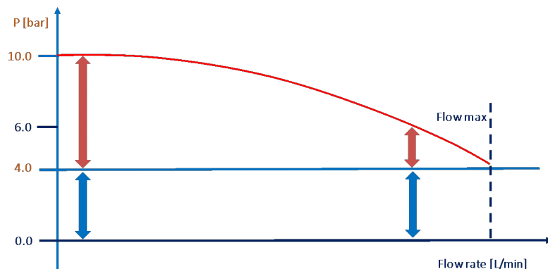
Abb. 55: Schaubild Systemdruck
