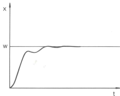
Abb. 80: Regelparameter X_p zu klein
