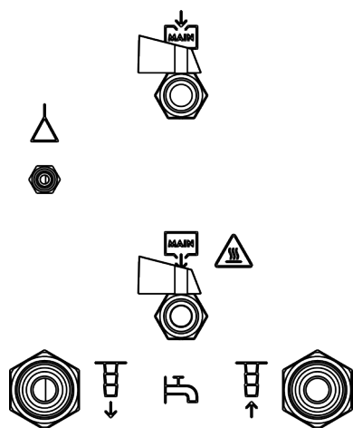
Abb. 35: Anschlussstutzen am Integral IN 2040 PW, IN 2050 PW
