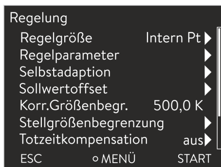
Abb. 45: Menü Regelung
