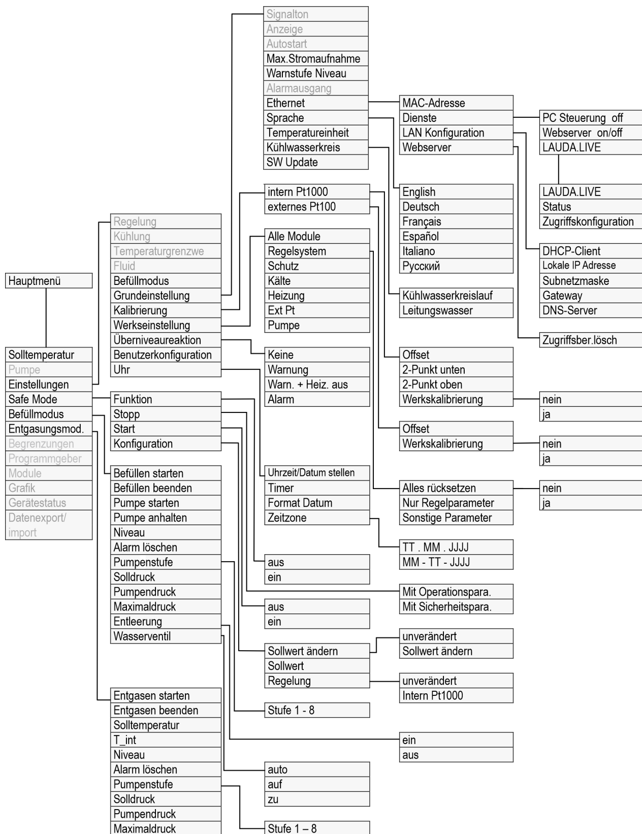
Abb. 38: Menü Teil 2, Fortsetzung von vorheriger Seite
