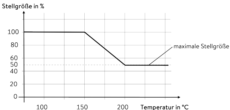
Abb. 47: dynamische Heizungsbegrenzung
