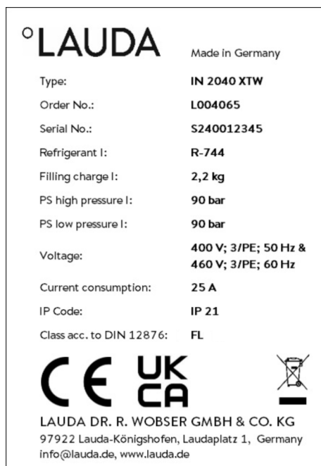
Abb. 10: Typenschild (Beispiel)
