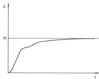
Abb. 82: Regelparameter T_n und T_v zu groß
