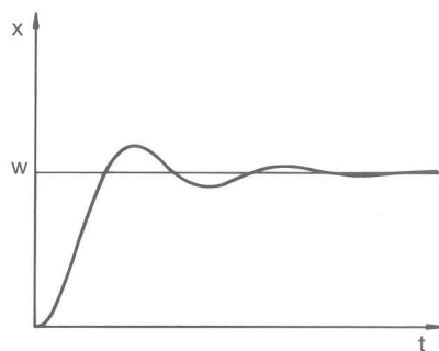
Abb. 81: Regelparameter T_n und T_v zu klein
