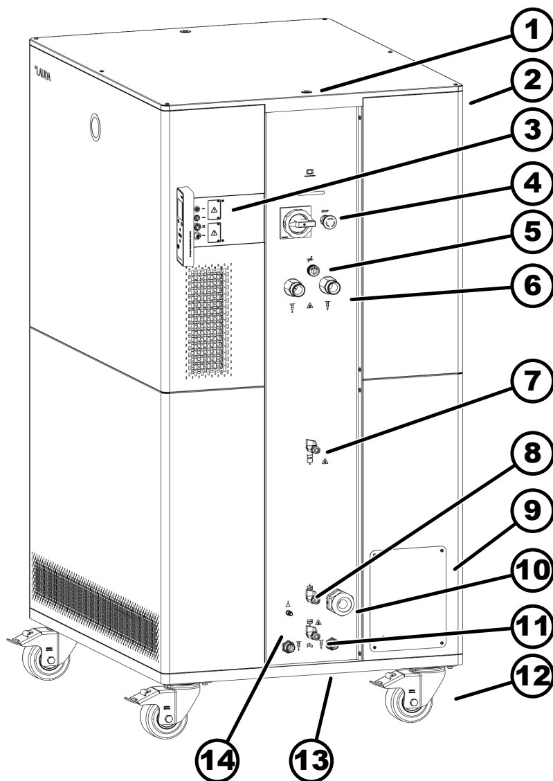
Abb. 6: Ansicht Integral IN 3540 XTW
