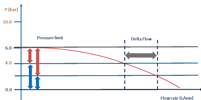
Abb. 56: Schaubild Systemdruck
