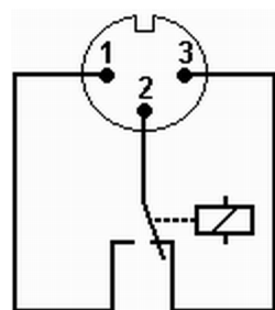
Abb. 15: Flanschstecker (Front) im Störungszustand
